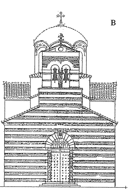
Αρχιτεκτονικά σχέδια του ναού: Α. βόρεια πλευρά, Β. πρόσοψη, Γ. ανατολική πλευρά.
